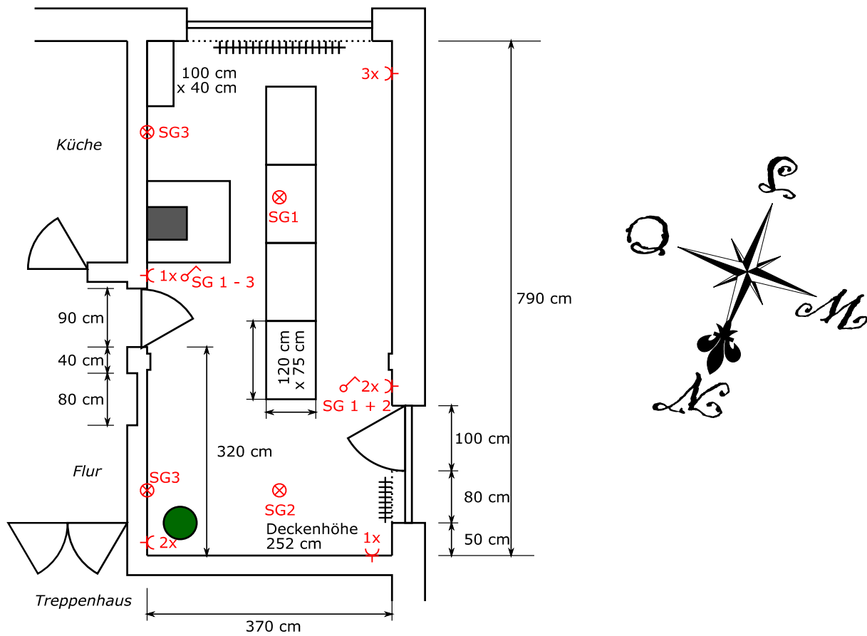
Grundriss 1: Status Quo, inkl. Einrichtung und Elektro
