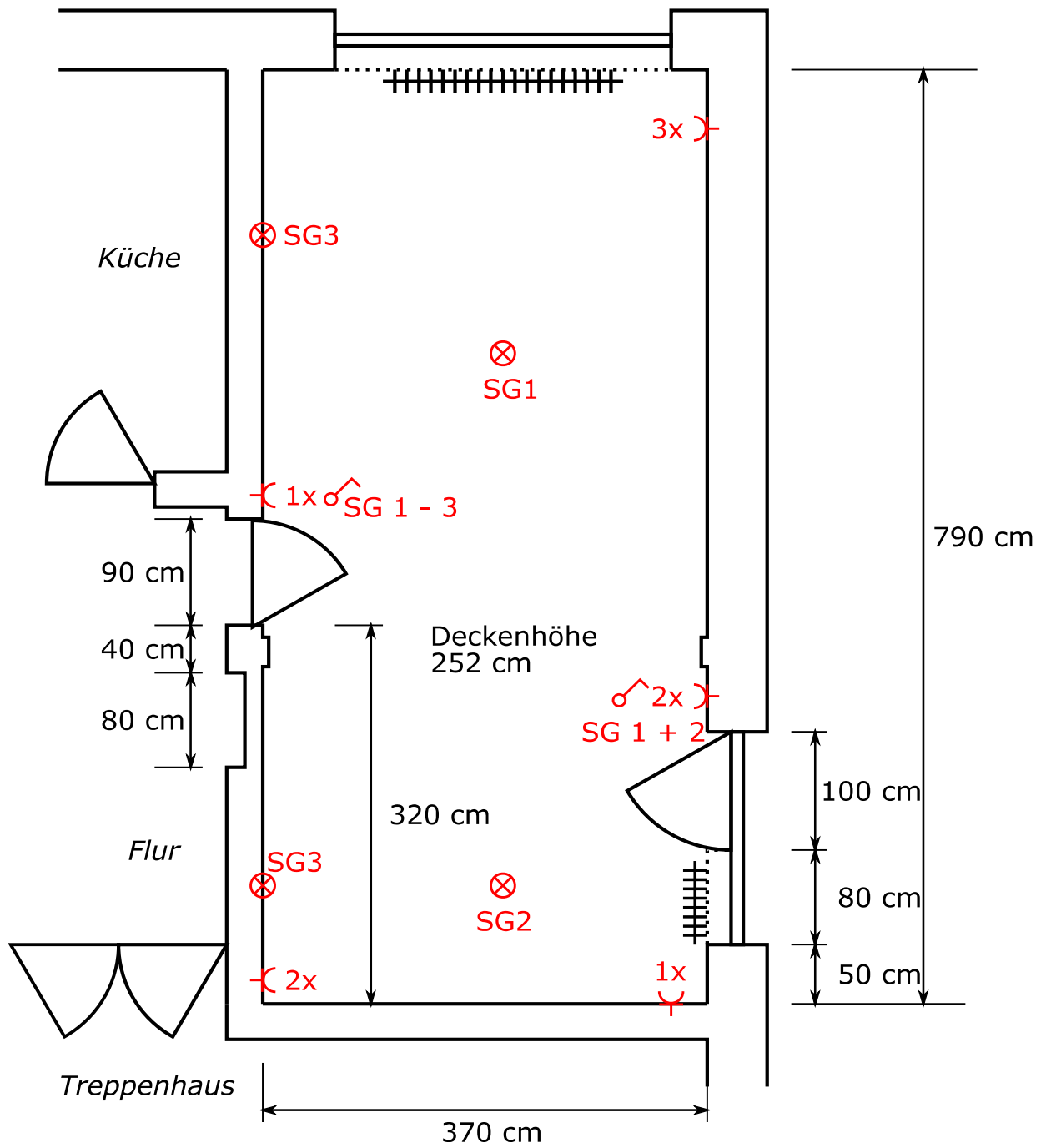
Grundriss 2: ohne Einrichtung, mit Bemaßung und Elektro
